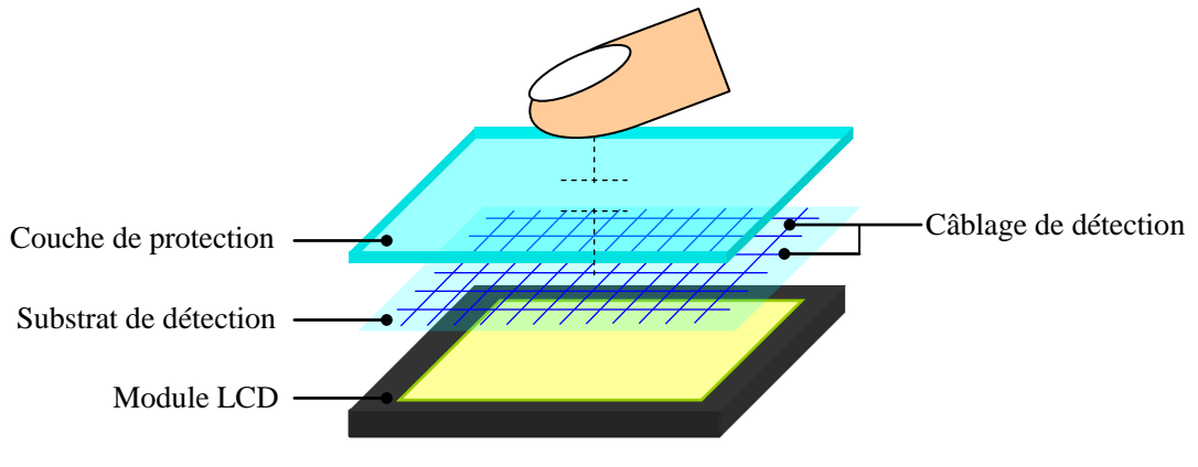
Image simplifiée d'une dalle tactile PCAP TFT-LCD
